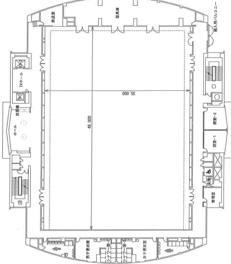
小アリーナ2F平面図 S=1/300 (atA3)
